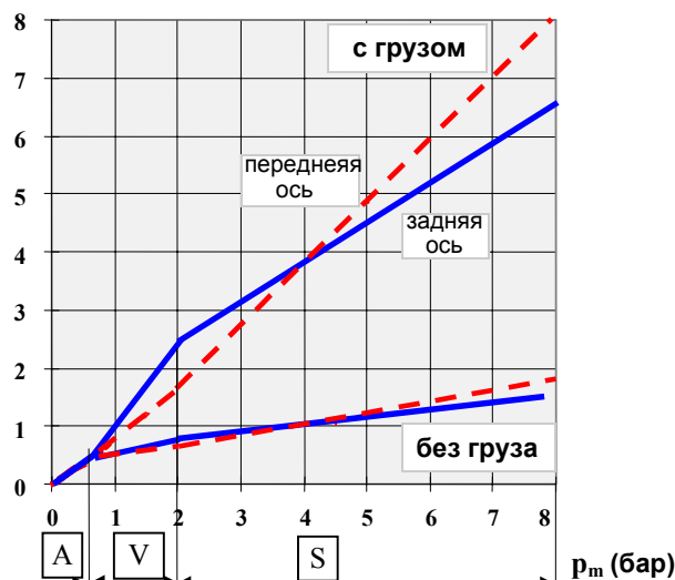
Распределение тормозной силы в прицепах с дышлом
