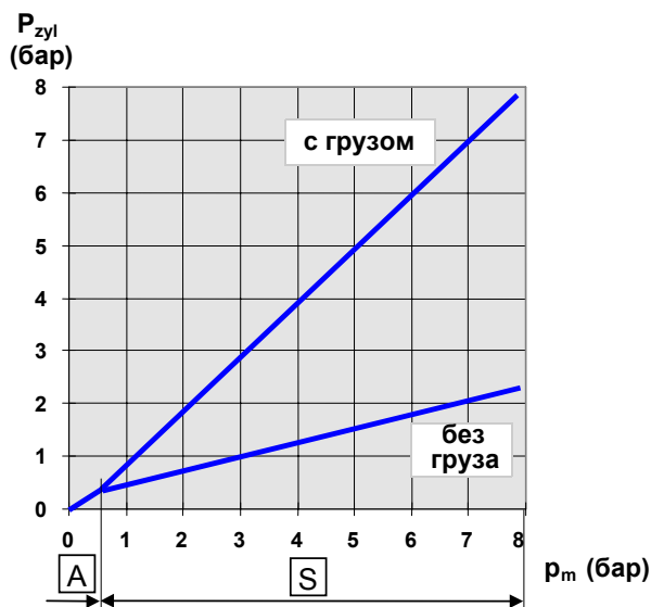
Функция SLV в полуприцепах
