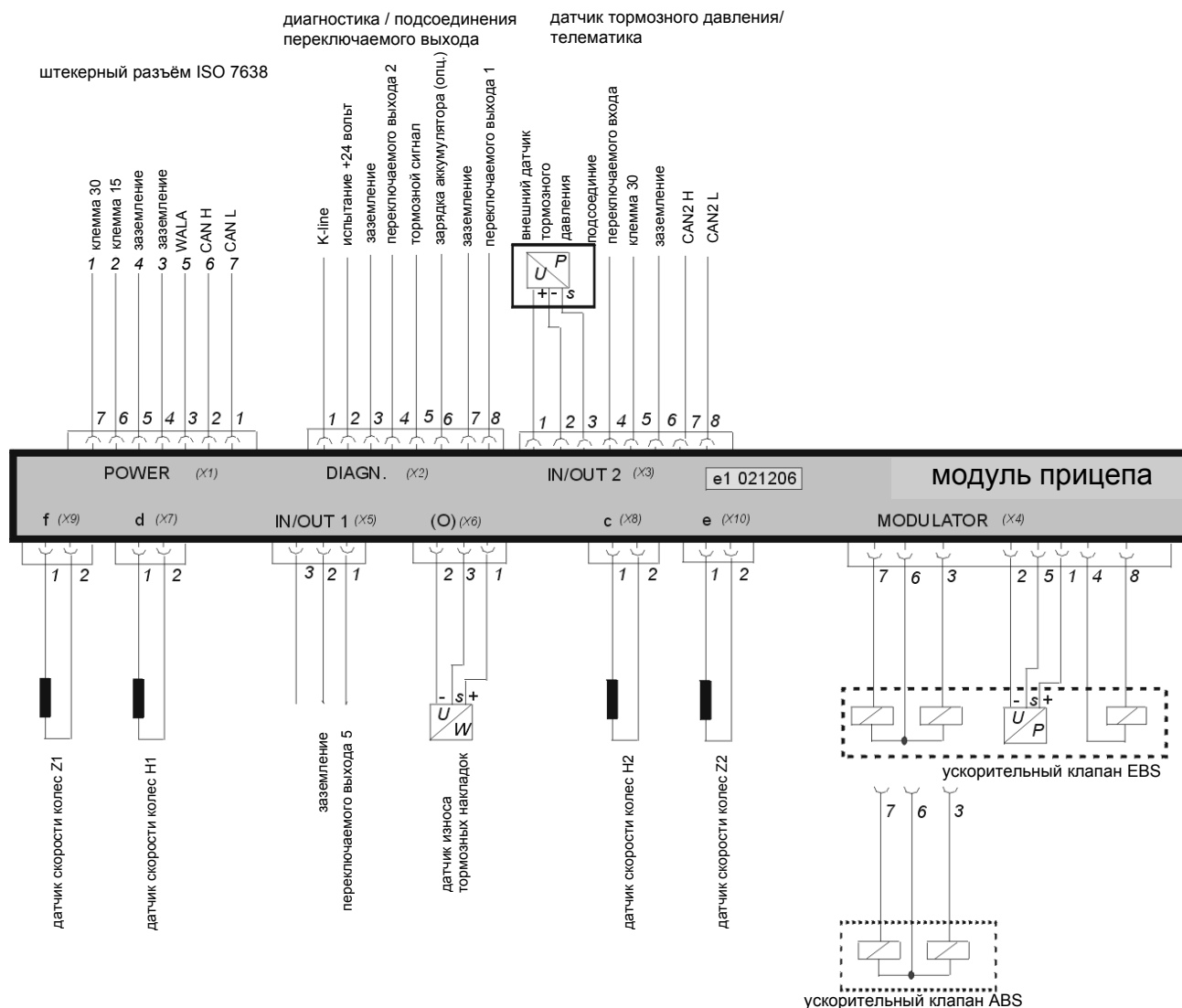
Рис 2. структура электрической/электронной системы
