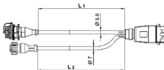
Диагностический кабель с соединением на клапан подъемной оси с одиночным контуром (3x0,5 2 ; 3x1,5 2 )
