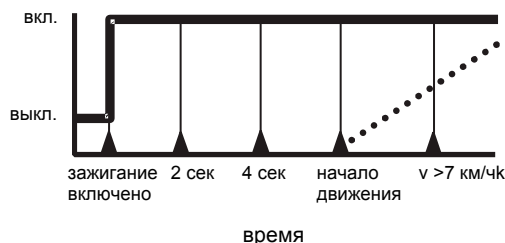
Последовательность предупреждающих сигналов, Случай В
