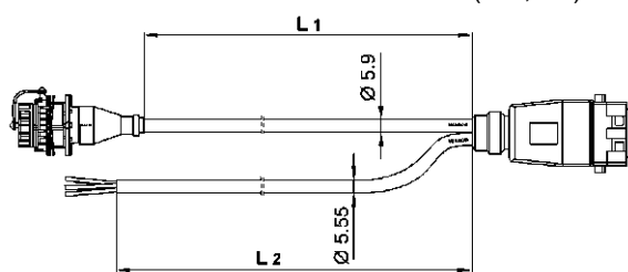
Диагностический кабель / ILS 1 + ILS 2 (3x0,75 2 )
