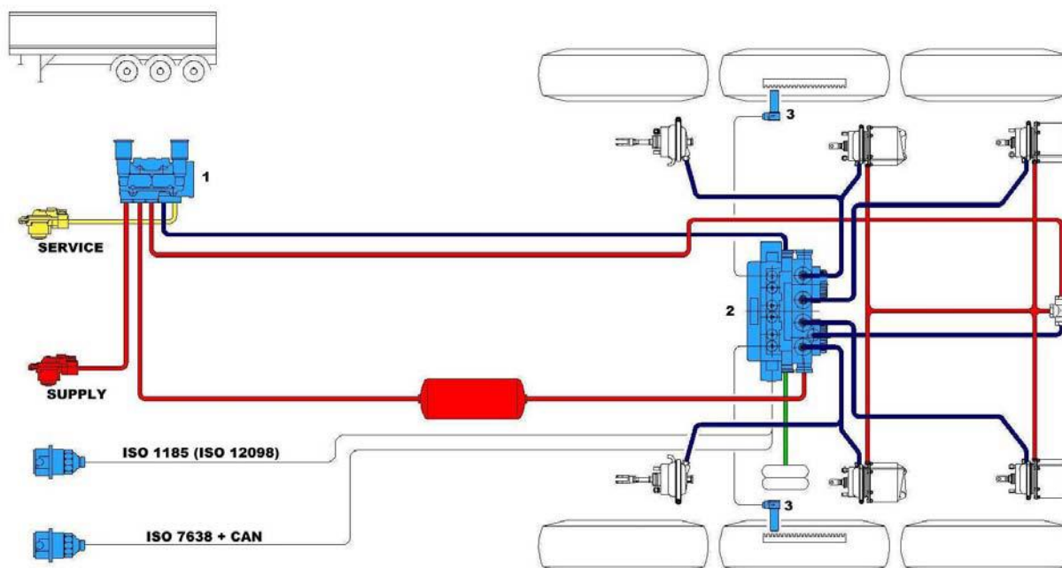
Рис 1. трехосный полуприцеп 2S/2M, оснащенный клапаном аварийного растормаживания
