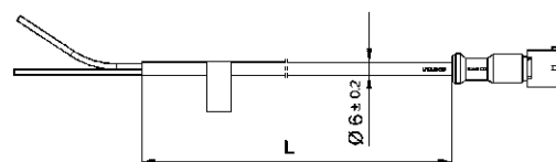
Кабель к кнопке активации функции вспомогательной тяги (модификация 150) тип вспомогательной тяги ВТ (2x0,75 2 )
