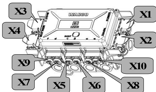
Рис 3. Электрические интерфейсы на модуляторе прицепа
