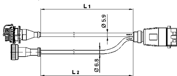
Диагностический кабель/ILS 1 с разъемом M27x1 (3x0,5 2 ; 2x1,5 2 )
