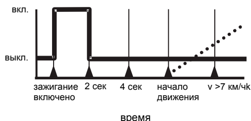
Последовательность предупреждающих сигналов, Случай А
