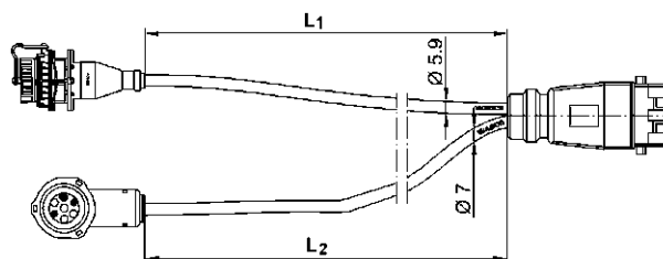
Диагностический кабель и кабель на модуль ELM (3x0,5 2 ; 3x1,5 2 )
